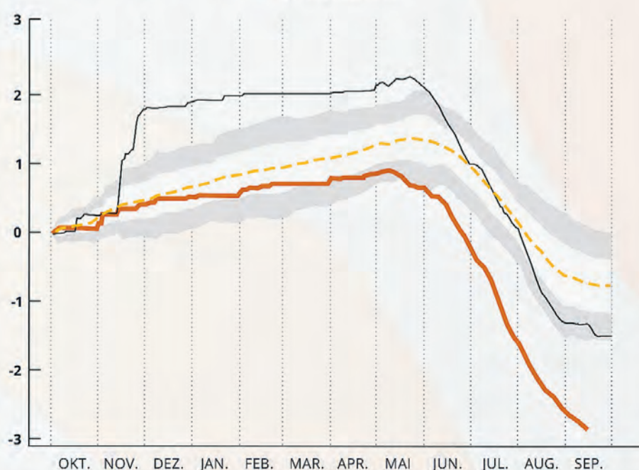
Die Grafik zeigt die Gletscherschmelze am Persgletscher im laufenden Jahr (rote Linie), im Hitzesommer 2003 (schwarze Linie) sowie als Durchschnitt der Jahre 2011 bis 2021 (gestrichelt).
